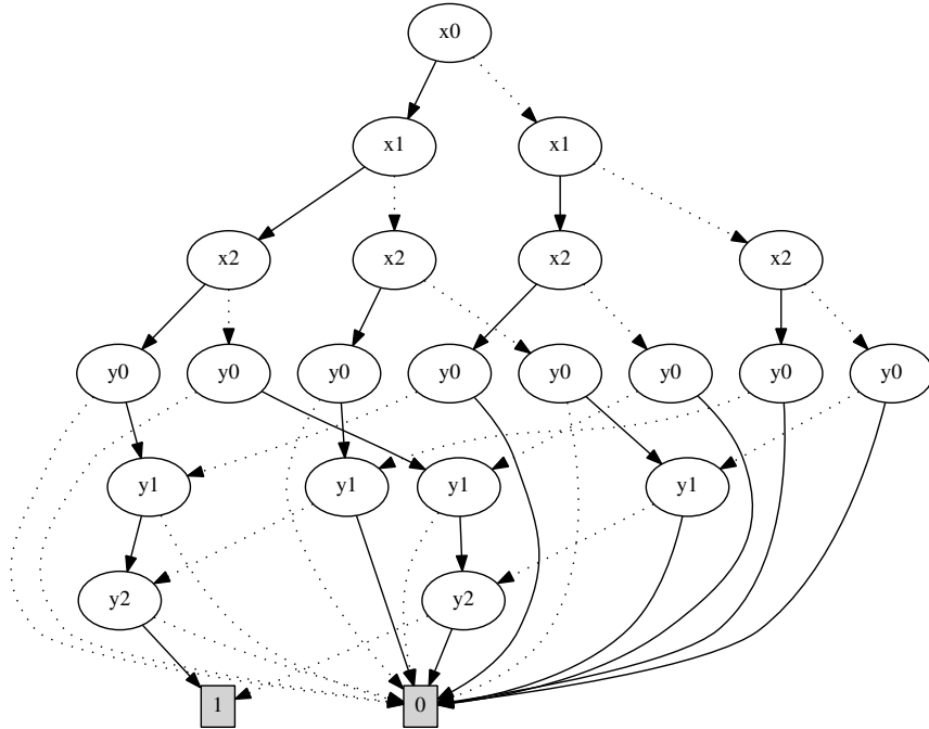
Abbildung 3: BDD der Funktion (x_0 \Leftrightarrow y_0) \wedge (x_1 \Leftrightarrow y_1) \wedge (x_2 \Leftrightarrow y_2) mit schlechter Variablenordnung
