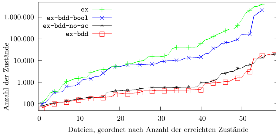
Abbildung 7: Quantilgraph der Dateien mit Anzahl der erreichten Zustände
