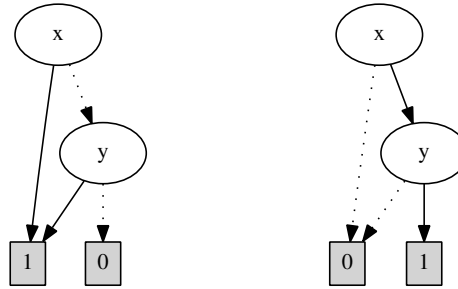
Abbildung 2: BDDs der Funktionen x \vee y und x \wedge y
