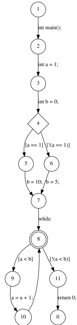
Abbildung 5: CFA zu Code 1
