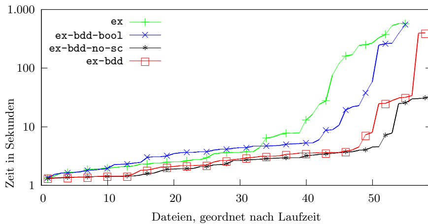
Abbildung 8: Quantilgraph der Dateien mit Laufzeit
