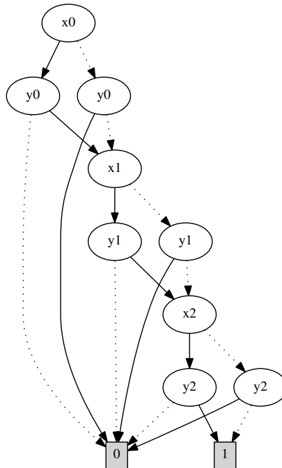
Abbildung 4: BDD der Funktion (x_0 \Leftrightarrow y_0) \wedge (x_1 \Leftrightarrow y_1) \wedge (x_2 \Leftrightarrow y_2) mit guter Variablenordnung
